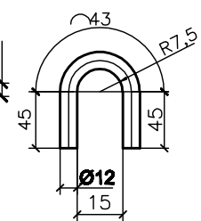
Поз.3
