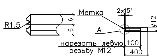
Узел А
