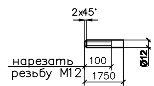
Поз.1
