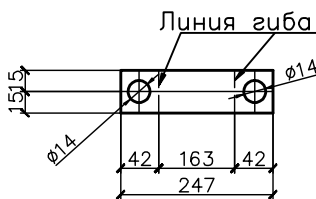
Развертка поз.5
